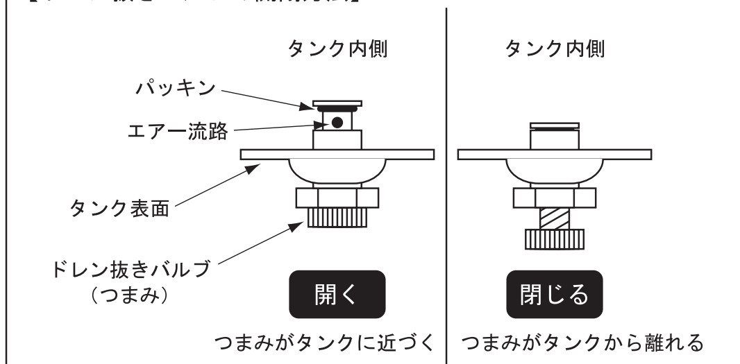
図1 各部の名称
